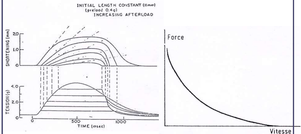
Relation Force-Vitesse isotonique
